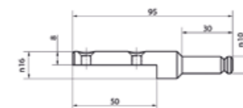
Halter für Laufschiene / Einhängeschiene
